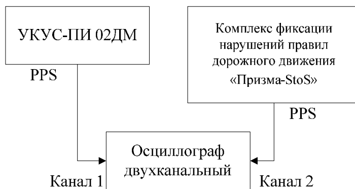
Рисунок 1 – Схема подключения
